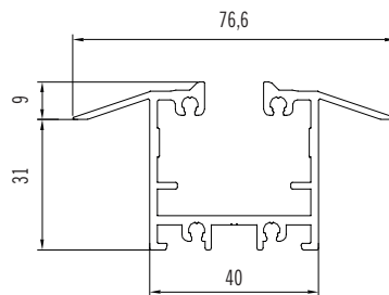
Perfil hoja 10mm Standard
