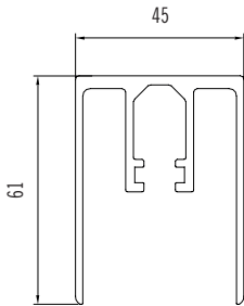
Perfil guía inferior inferior Standard
