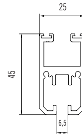
Perfil hoja 12mm Standard
