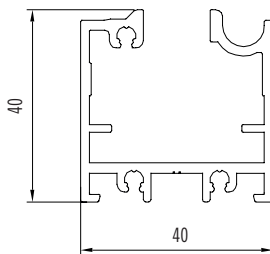
Perfil hoja 8mm Standard
