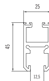
Perfil hoja 12mm Standard
