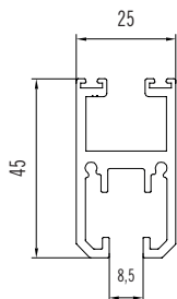
Perfil hoja 8mm Standard
