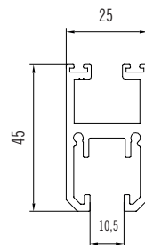
Perfil hoja 10mm Standard
